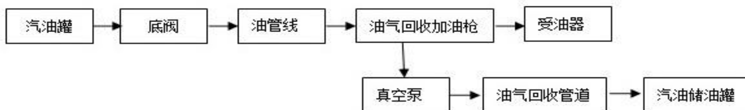
汽油加油工艺流程简图：
